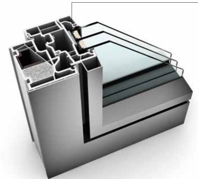
I-tec Verglasung
